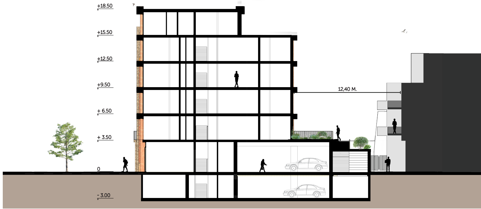
Doorsnede A
