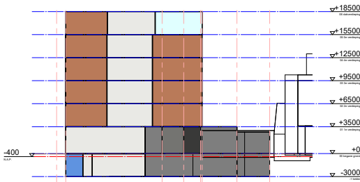
Doorsnede
