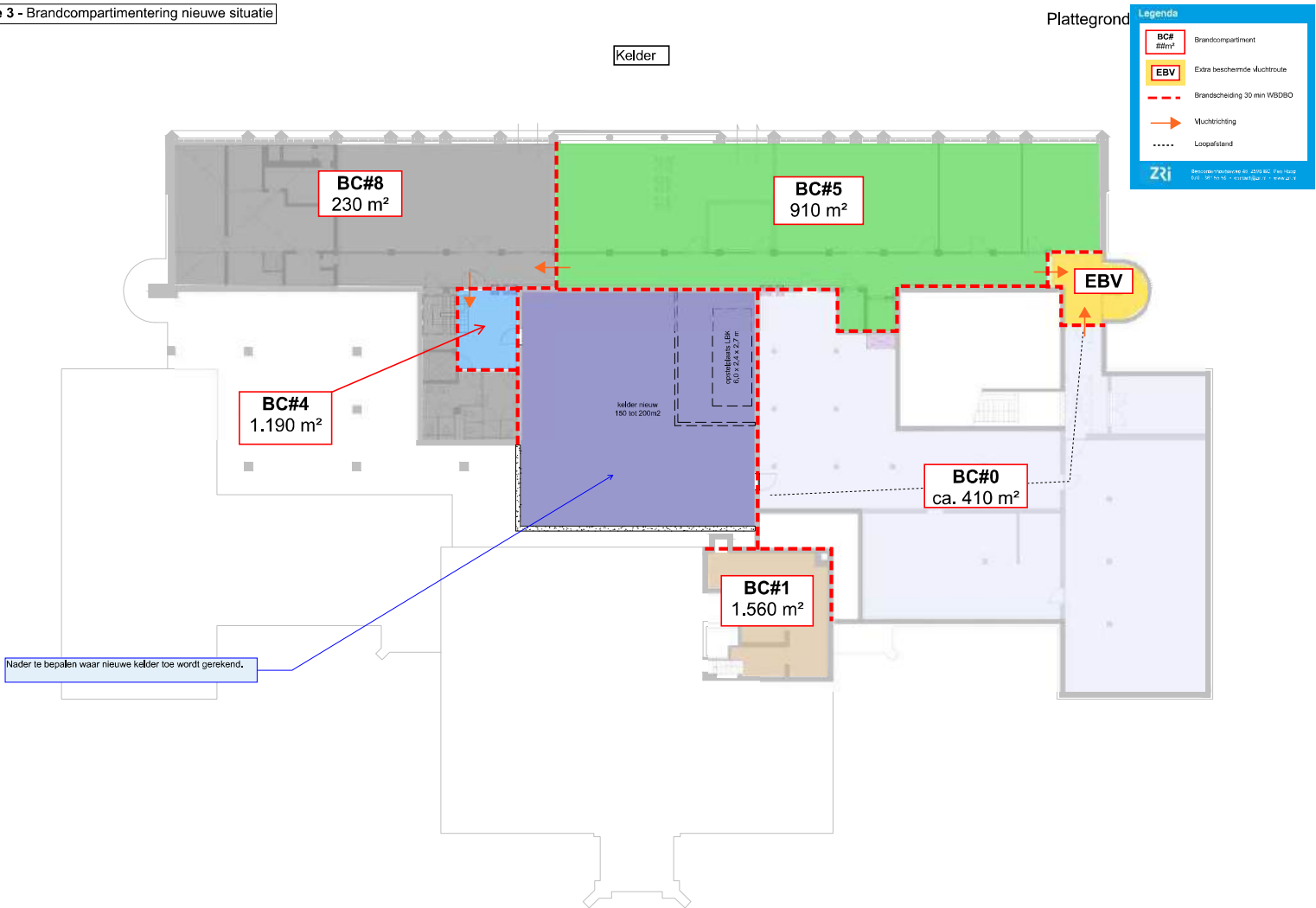
Bijlage 3 - Brandcompartimentering nieuwe situatie
